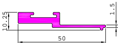
S5239 0.443 kg/m
