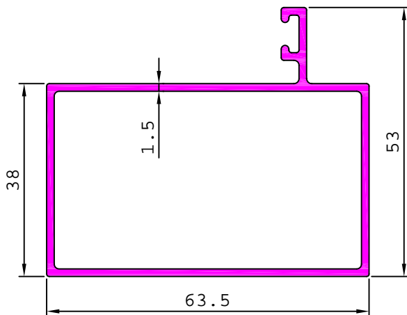
S5232 0.901 kg/m
