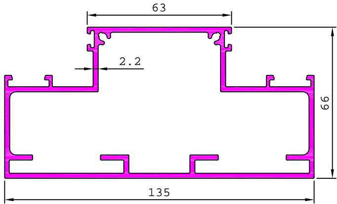
S6178 2.905 kg/m
