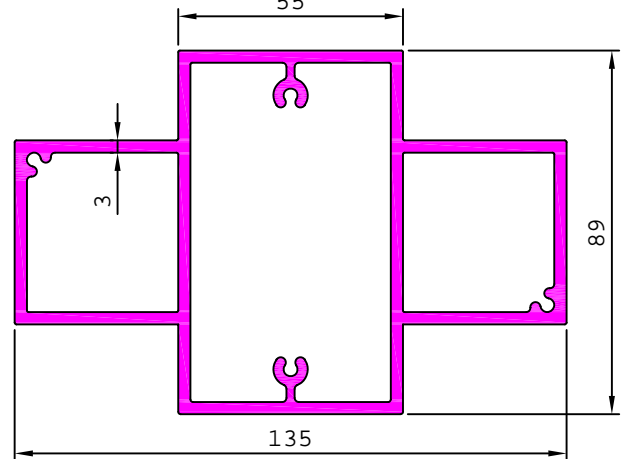
S6181 4.479 kg/m
