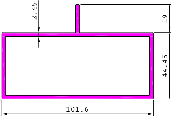
20141 1.992 kg/m
